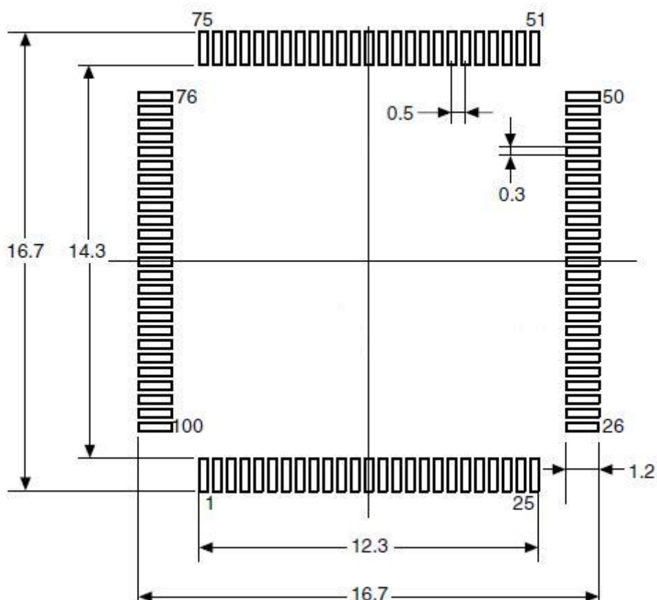
图 20 LQFP100 - 100 引脚，14 x 14mm 焊接 Layout 建议
