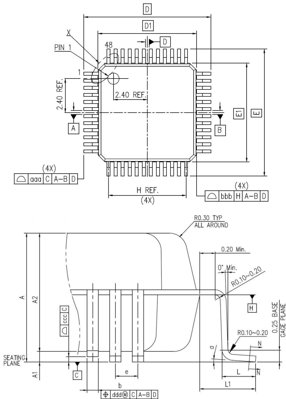
图 23 LQFP48 封装图
