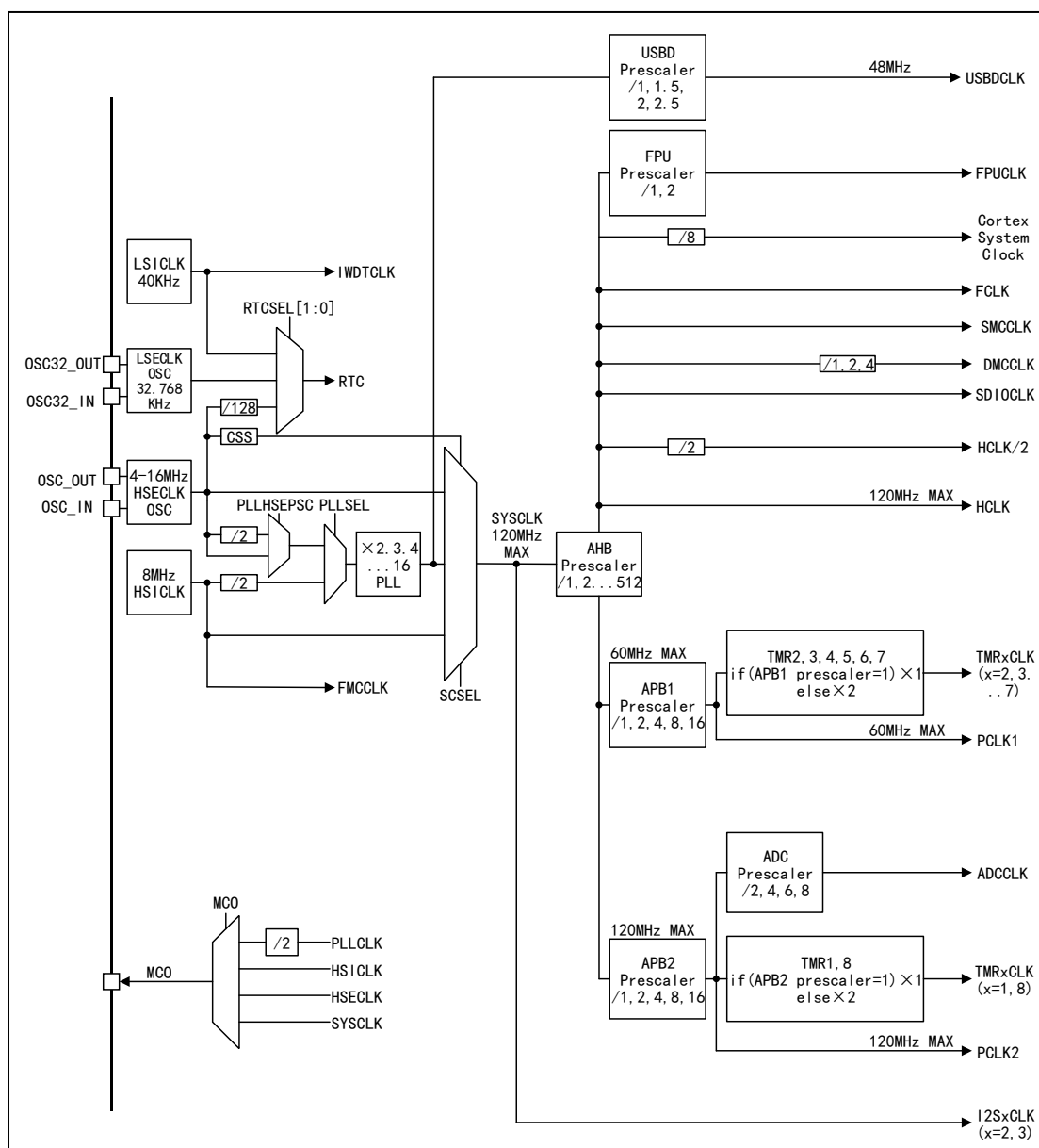
图 7 APM32E103xCxE 时钟树
