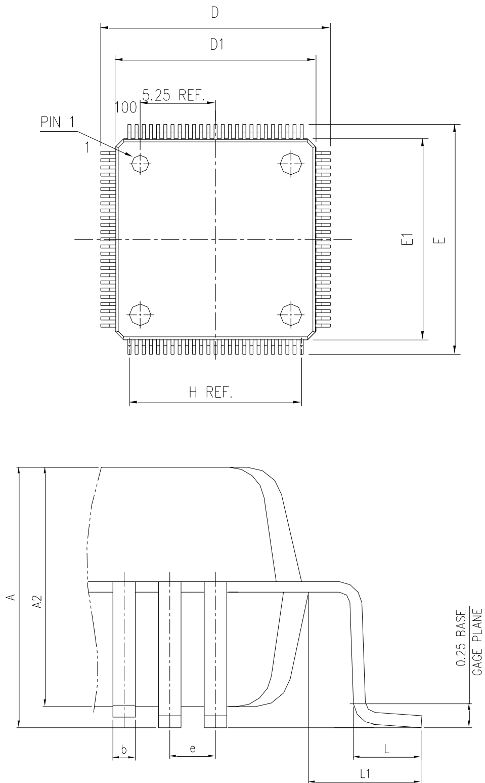
图 19 LQFP100 封装图
