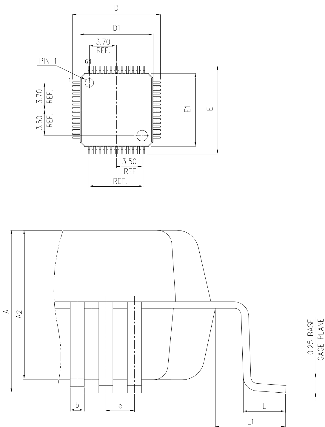
图 21 LQFP64 封装图
