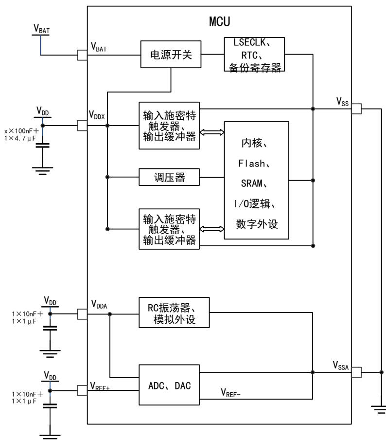
图 8 电源方案
