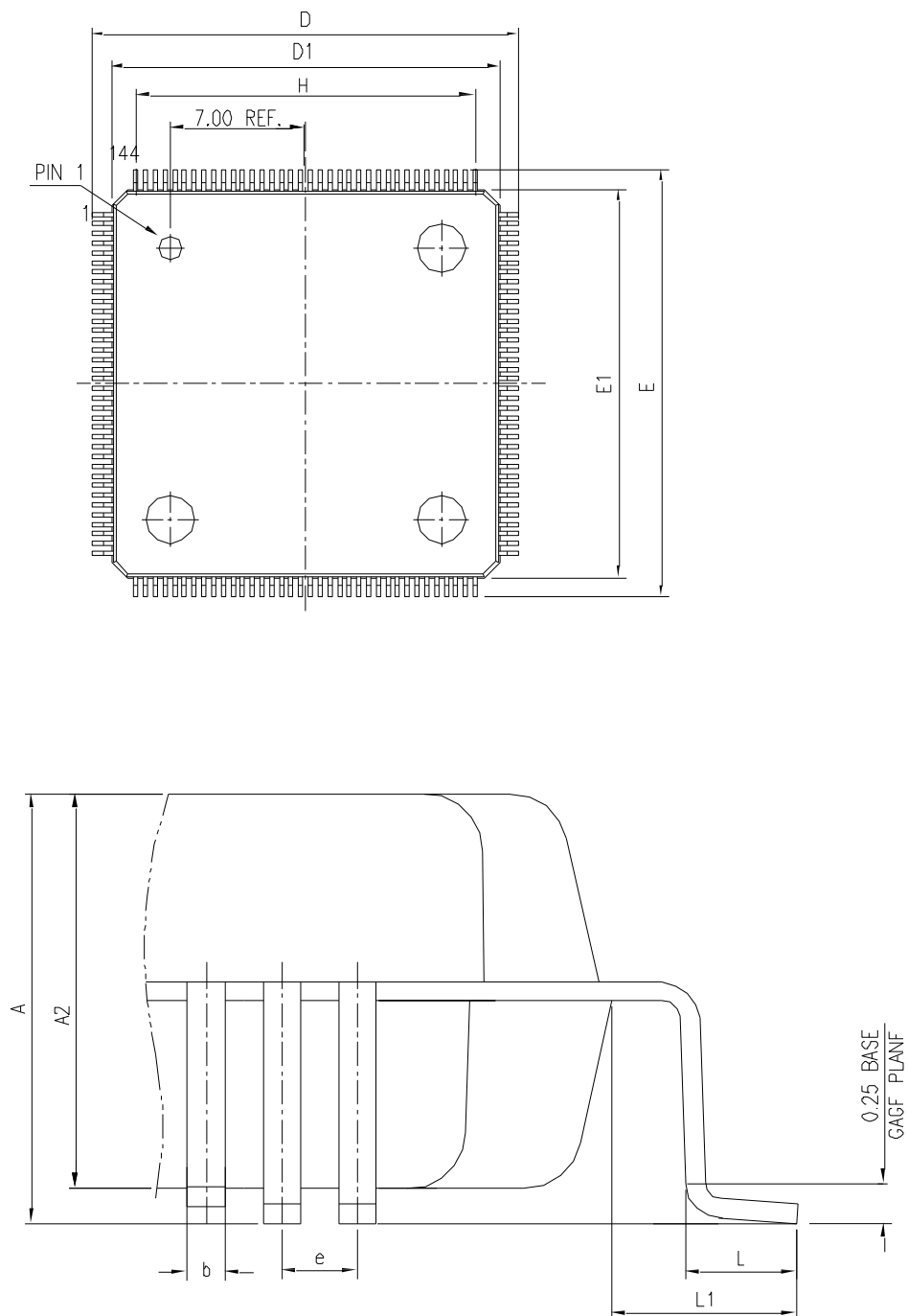
图 17 LQFP144 封装图
