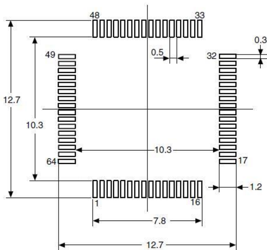
图 22 LQFP64 - 64 引脚，10 x 10mm 焊接 Layout 建议
